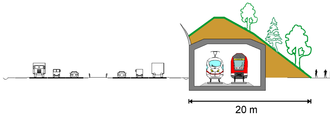
Abb. 7: Vermaßter Querschnitt 6-spurige Autobahn mit Lärmschutz-Tunnel in Lärmschutzwall an Engstellen (minimaler Flächenbedarf)
