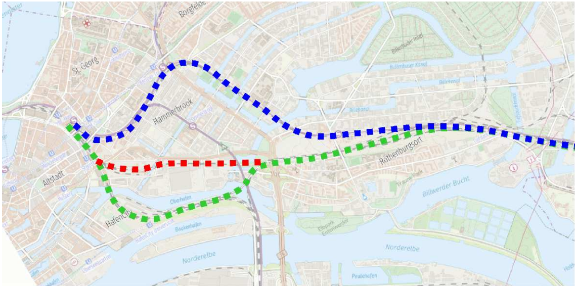
Abb. 8: Drei Gleistrassen von Hamburg Hbf in Richtung Moorfleet
